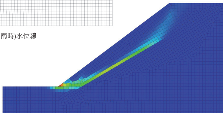
最大せん断ひずみ分布図(安全率=1.334)
