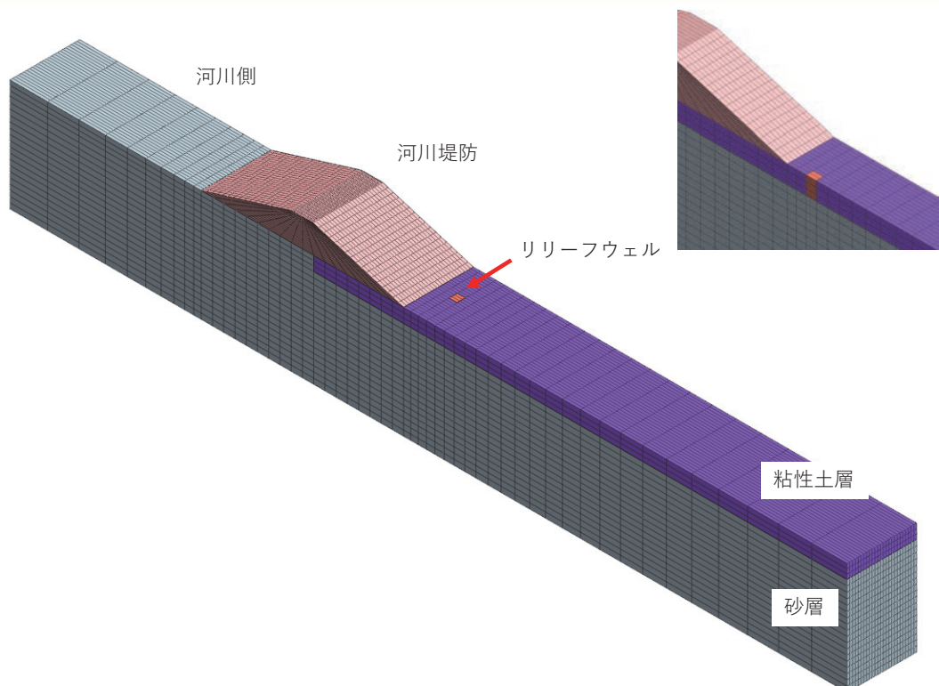
解析モデル図
