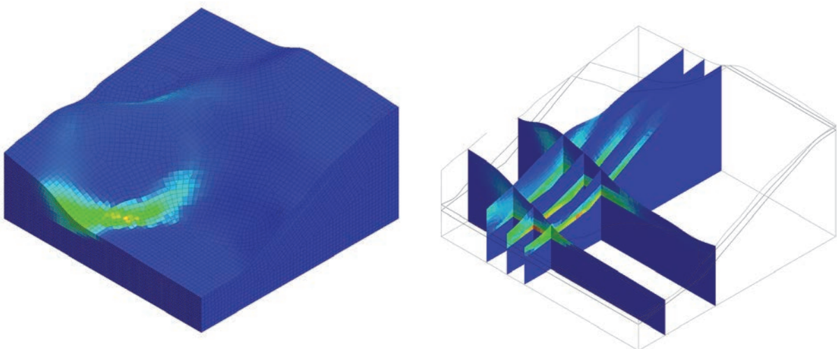
最大せん断ひずみ分布図
