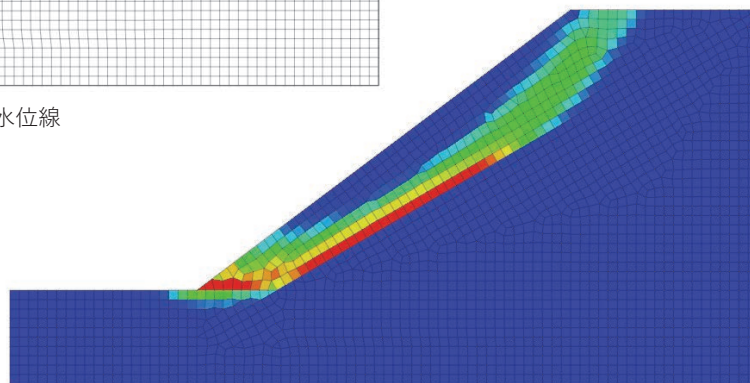
最大せん断ひずみ分布図(安全率=1.575)
