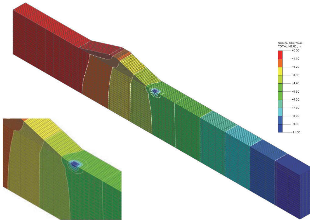
全水頭コンター図
