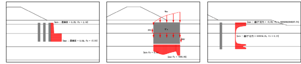
締りめ工法 固結工法 締りめ工法
