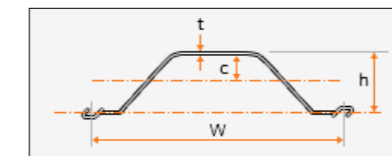
鋼部材使用工法
