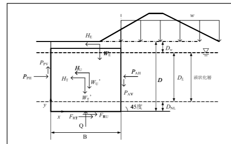
固結工法の自重計算
