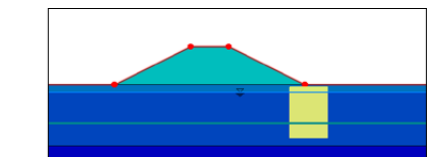
固結工法
