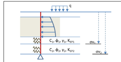
鋼部材の土水圧計算
