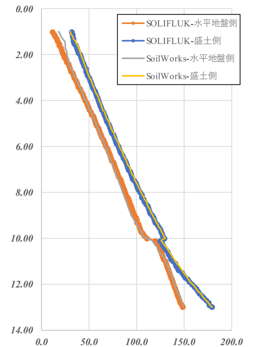
土圧の比較結果
