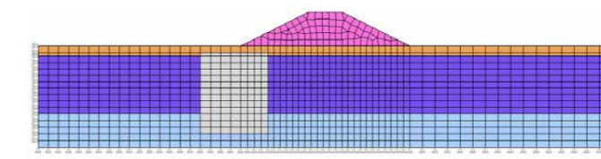
FEMモデル(SoilWorks地盤応力モジュール)
